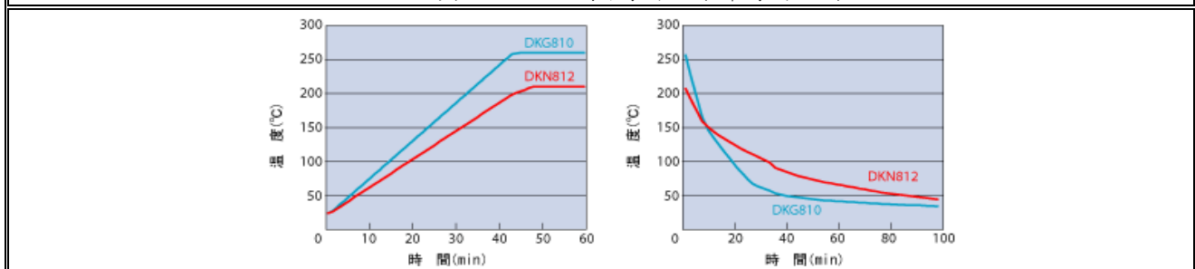
DKG810 與 DKN812 加熱時間，冷卻時間 比較
