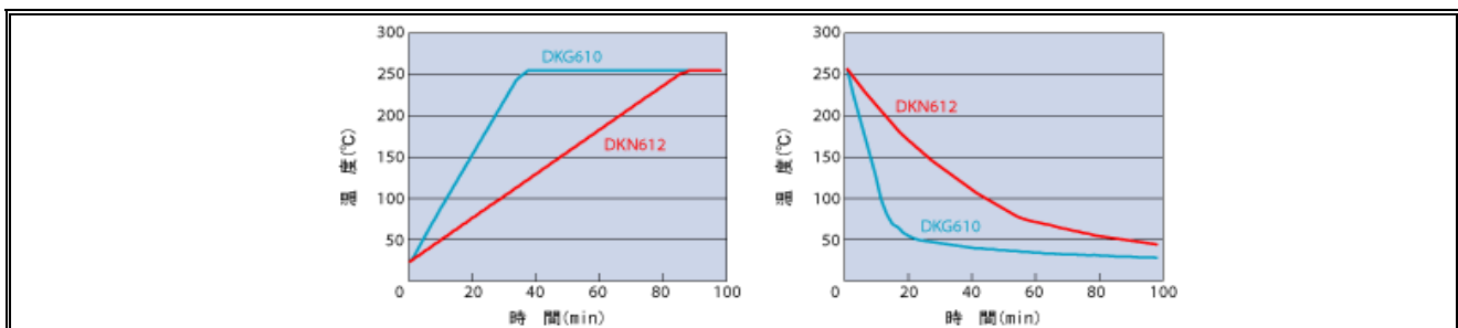
DKG610 與 DKN612 加熱時間，冷卻時間 比較
